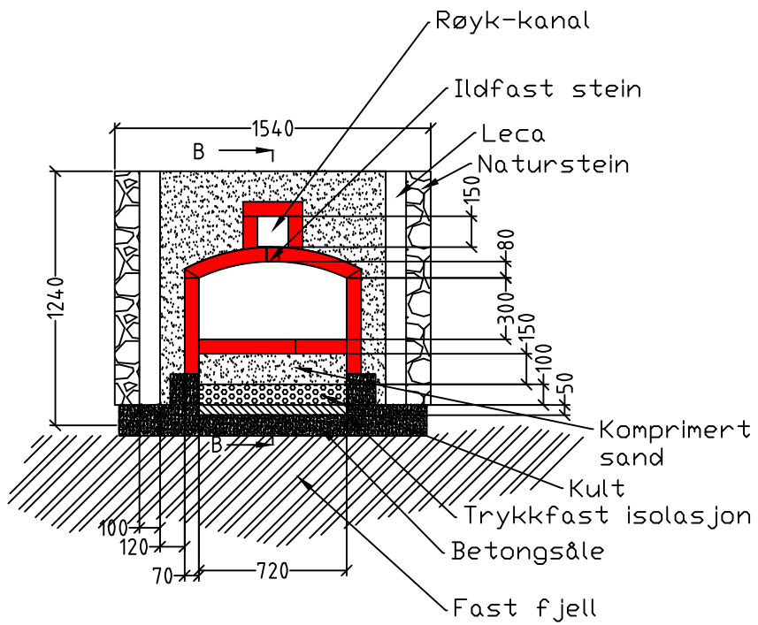
Snitt A-A
